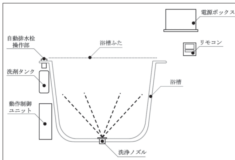
図2 各部の名称
