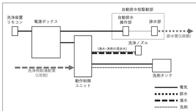
図1 自動浴槽洗浄システムの例
