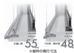
※縦枠の奥行寸法
