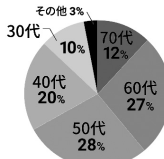
図4 年代
