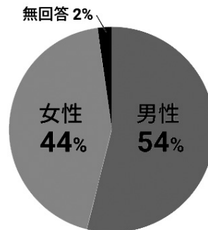
図3 性別
