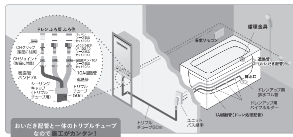
ドレンアップ方式システム図
