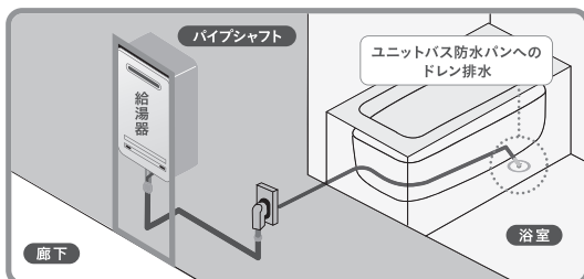
ドレンアップ方式による排出方式のイメージ図
